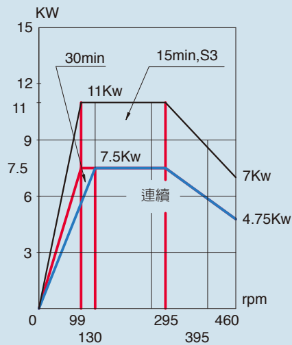
低速檔扭力圖 (Low Gear)
