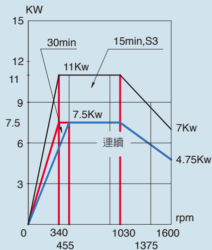
高速檔扭力圖 (High Gear)
