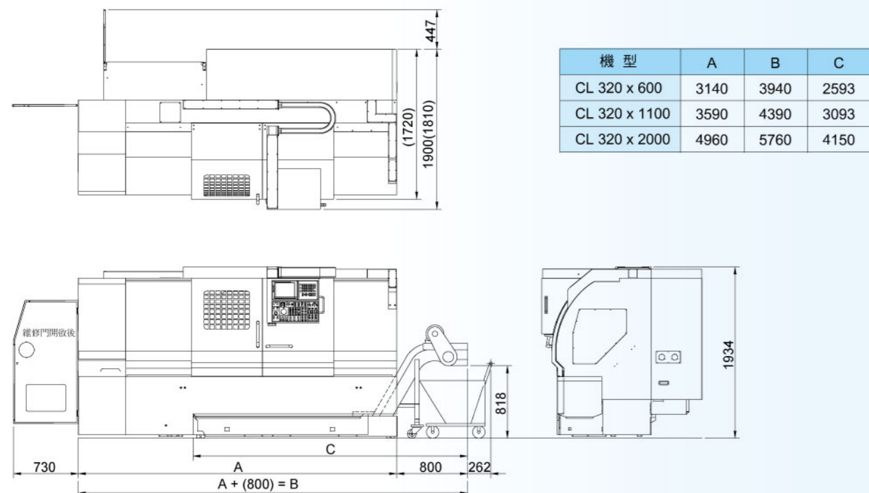
機械外型圖 Dimensional Drawing (mm)
